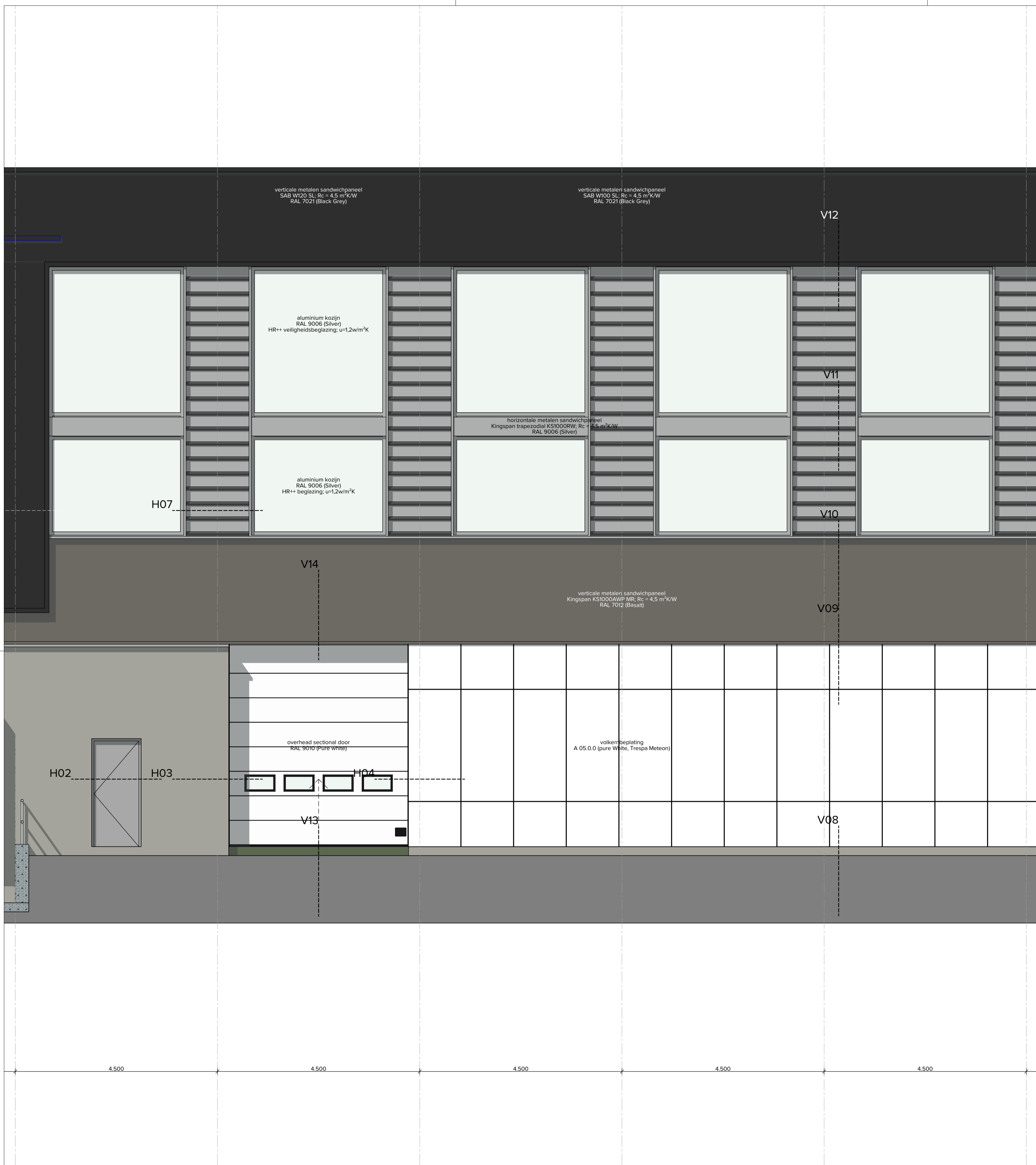
Voorgevel 1
