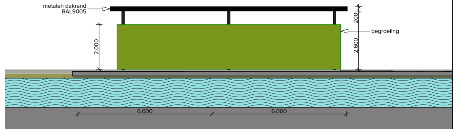
Achteraanzicht Bicycles
